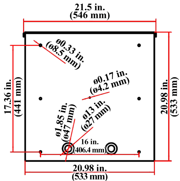
BOTTOM
