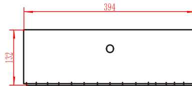
FRONT DOOR
